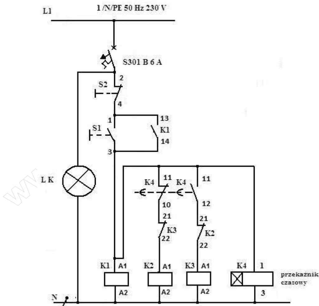
Rys.1. Schemat układu sterowania rozruchem gwiazda – trójkąt silnika indukcyjnego 3-fazowego.
