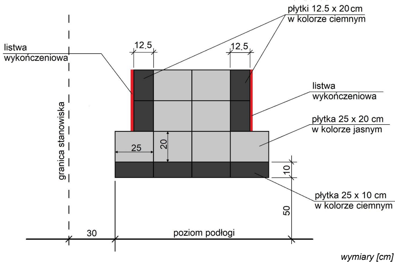
Widok okładziny z płytek ceramicznych
