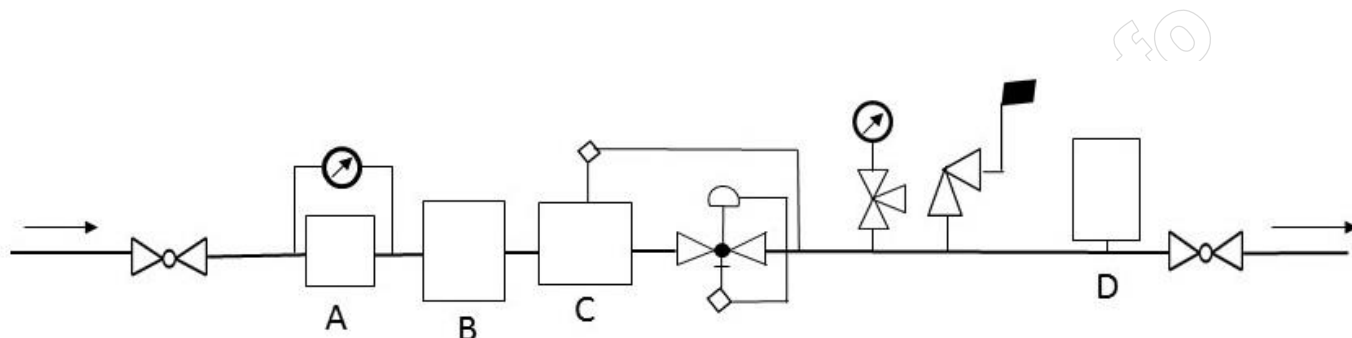
Rysunek 3. Schemat ciągu redukcyjnego sieci gazowej
