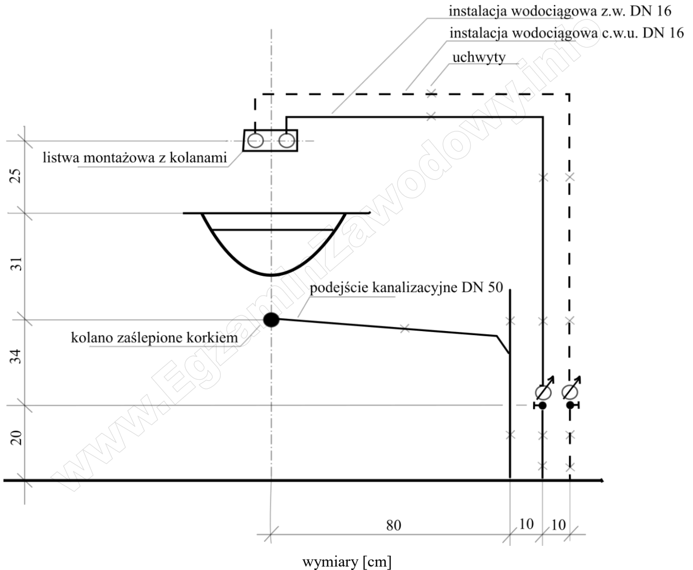
Rysunek. Widok instalacji wodociągowej i kanalizacyjnej.
