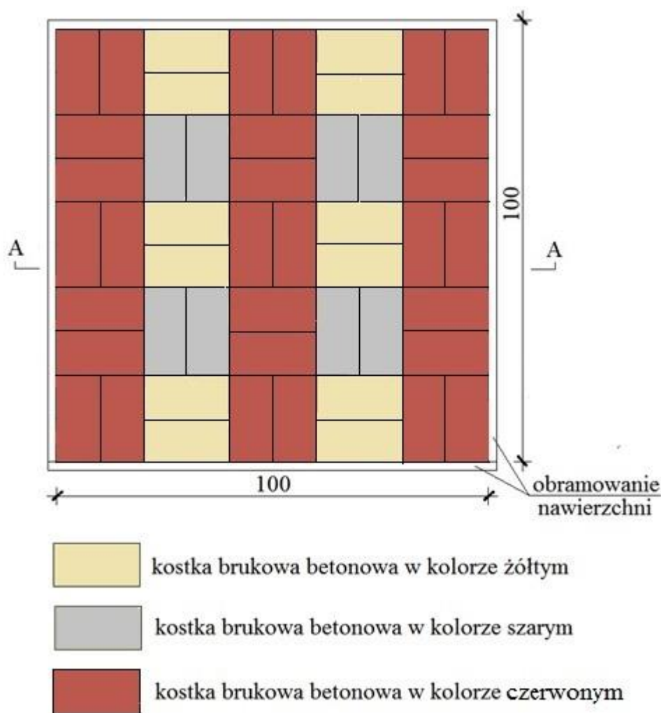
Rysunek 1. Rzut poziomy fragmentu nawierzchni do ułożenia
