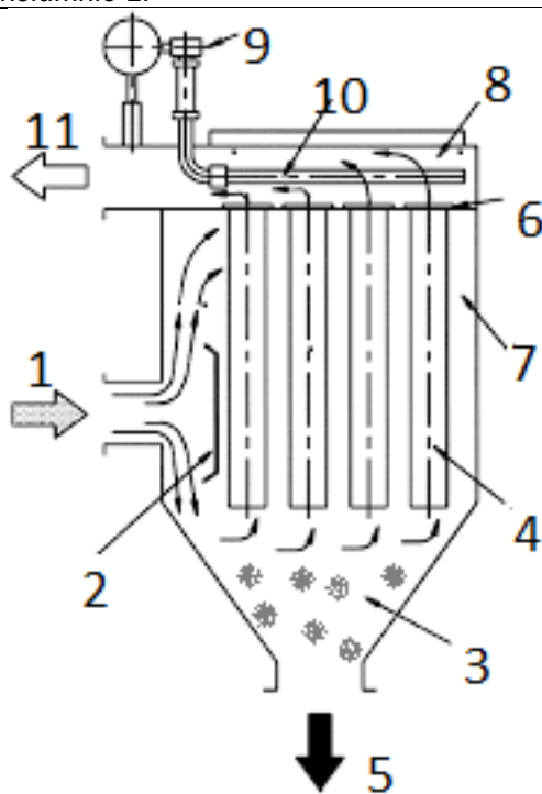
Schemat budowy odpylacza workowego
