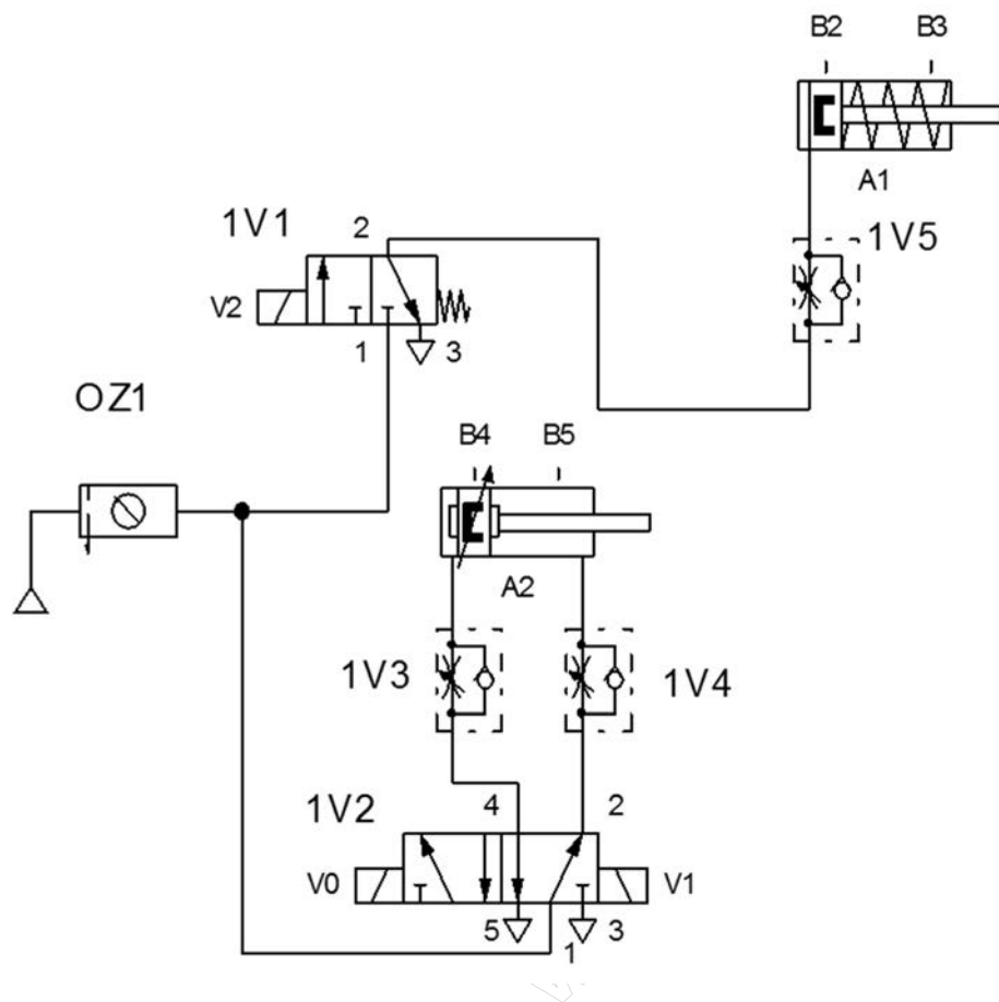
Schemat połączeń pneumatycznych
