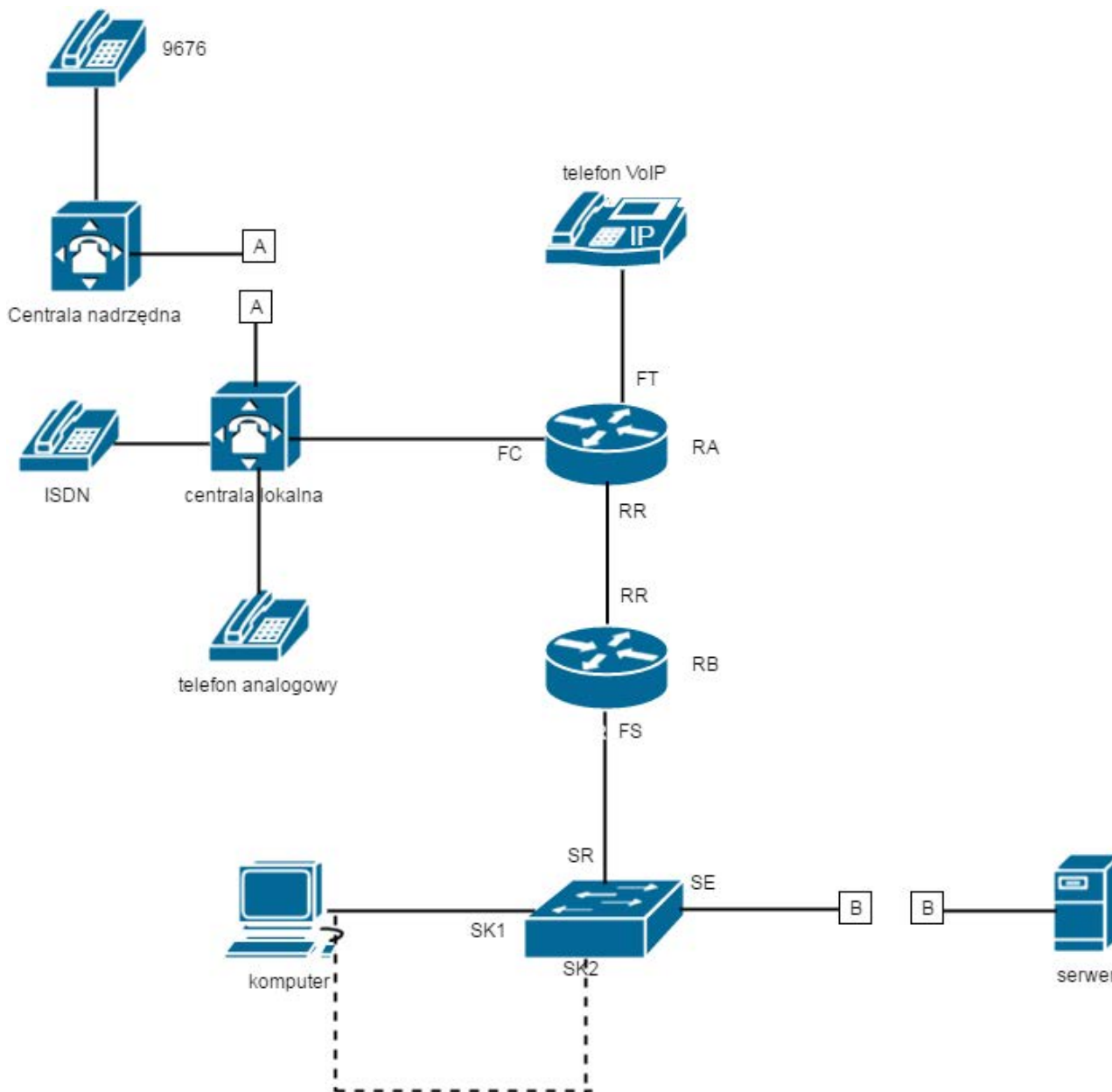
Rys.1. Schemat usytuowania urządzeń w sieci teleinformatycznej
