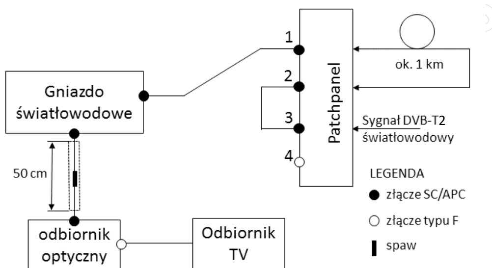
Schemat połączeń instalacji antenowej
