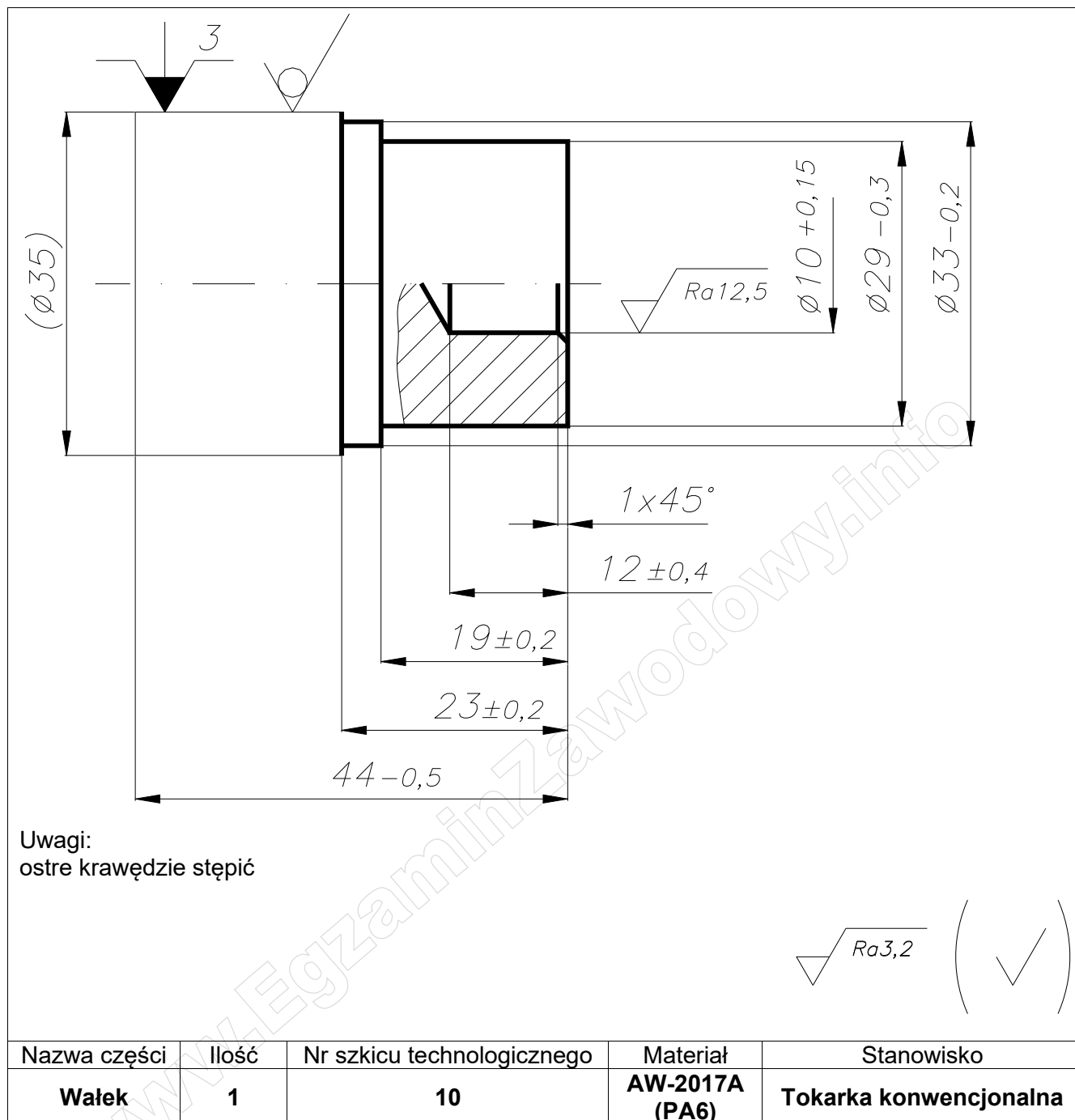
Szkic technologiczny do operacji nr 10
