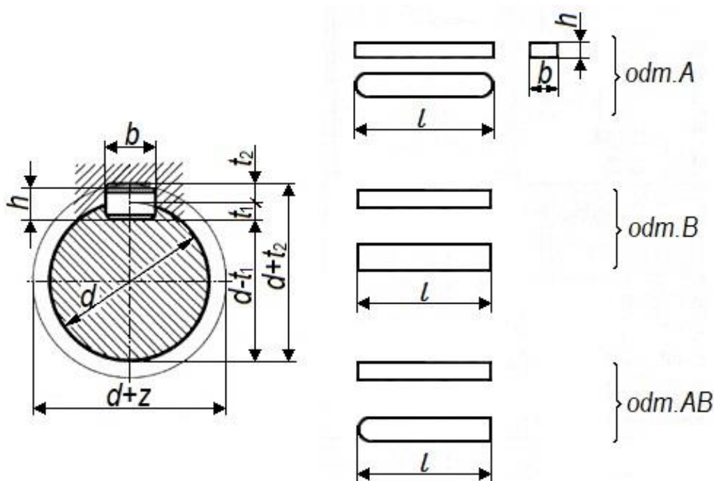
Dane do obliczeń połączenia wpustowego
