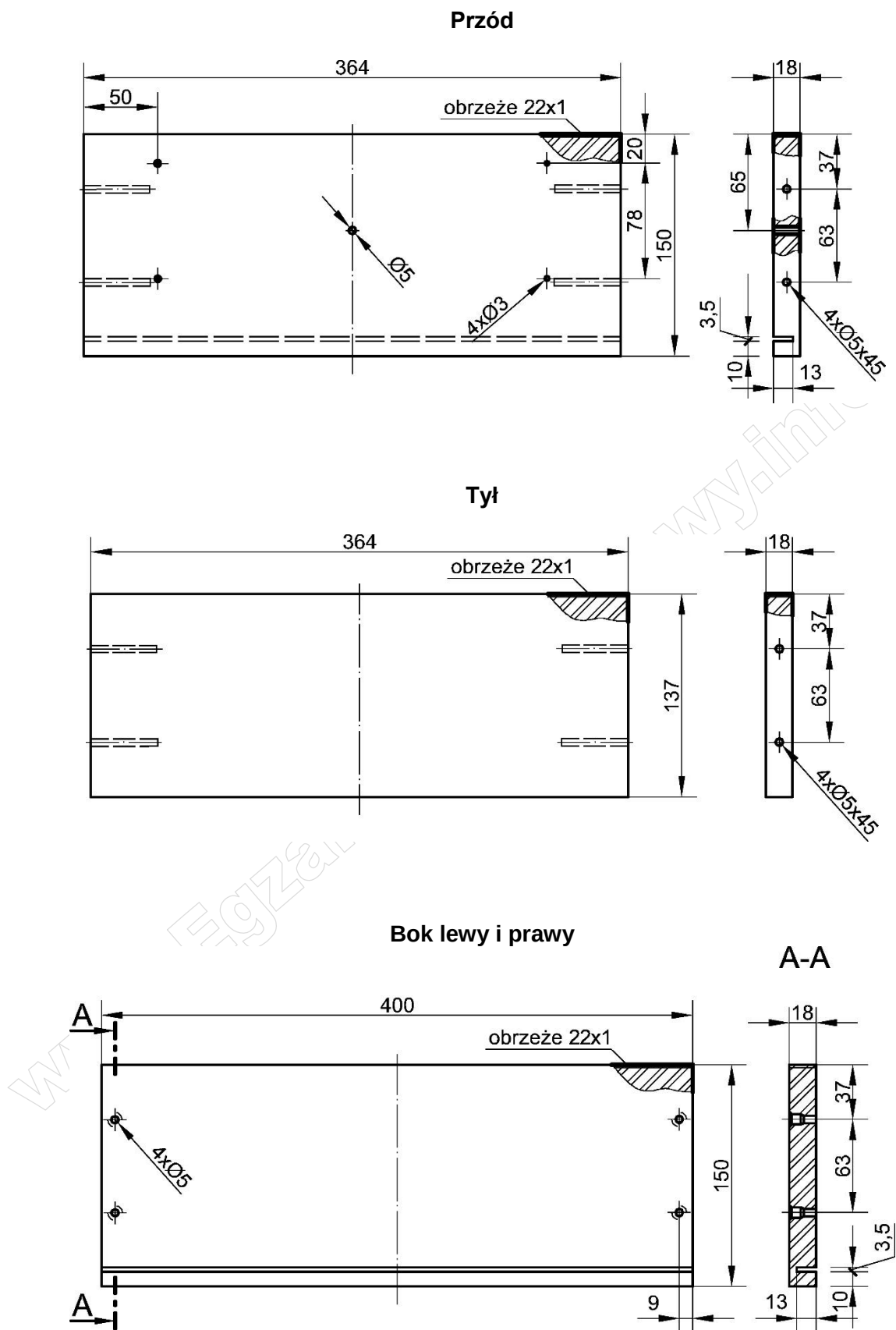
Rysunek 3. Elementy korpusu szuflady
