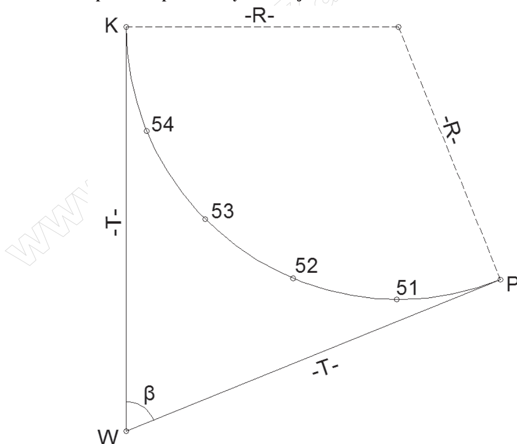
Układ punktów pomiarowych i wzajemne rozmieszczenie elementów łuku
