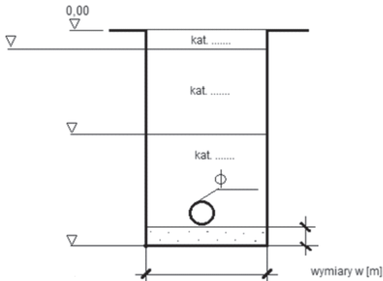
Rysunek 1. Przekrój poprzeczny wykopu pod kolektor sanitarny do zwymiarowania oraz uzupełnienia opisów: kategorii gruntu, rzędnych zalegania warstw gruntu i średnicy kolektora
