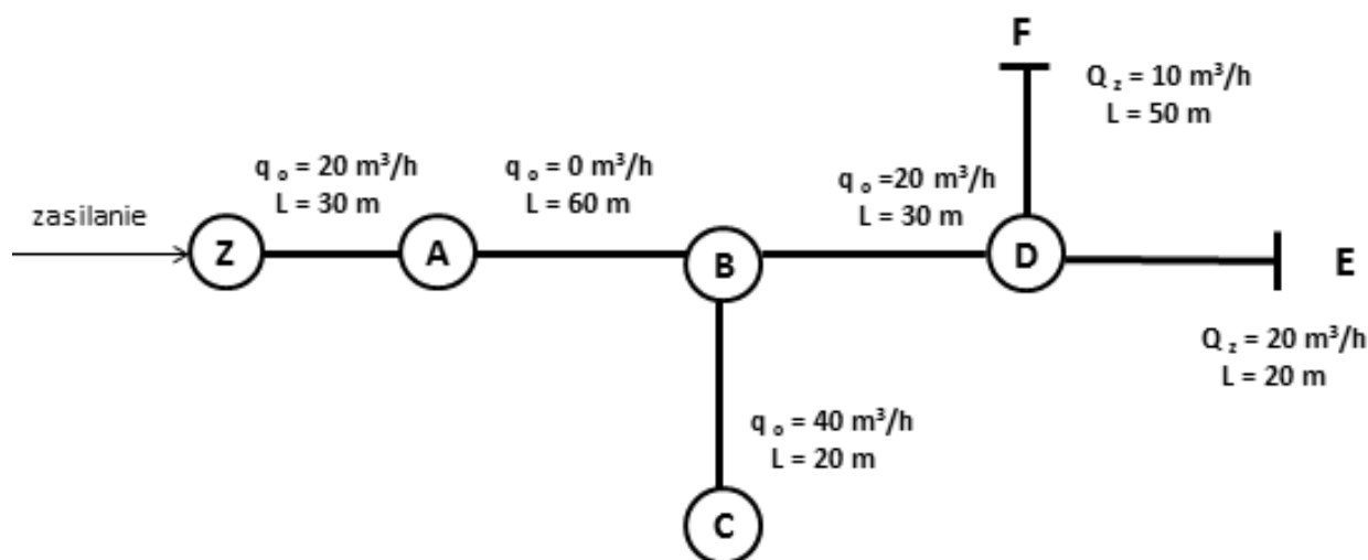
Rysunek 1. Osiedlowa sieć gazowa niskiego ciśnienia
