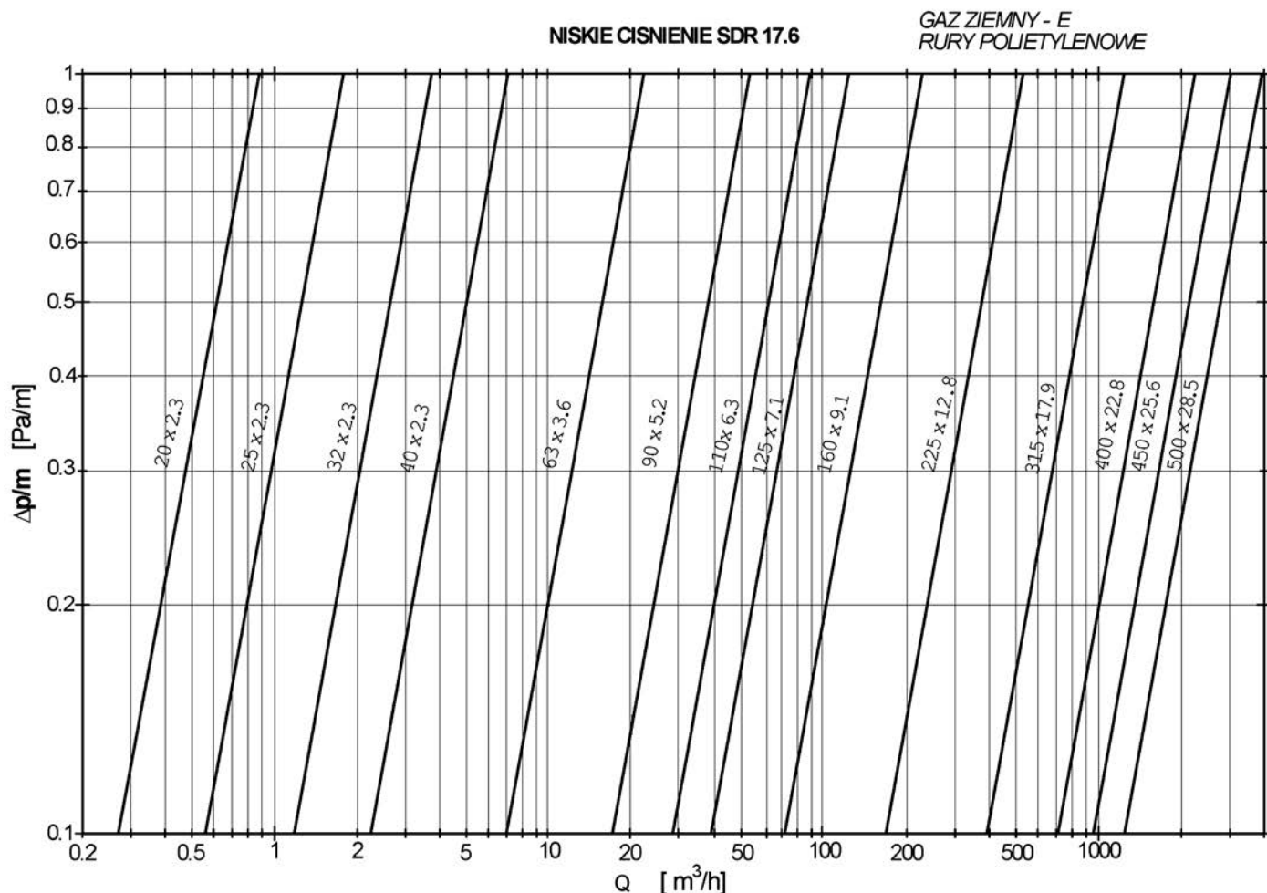
Nomogram. Dobór średnic rurociągów gazowych niskiego ciśnienia PE 100 SDR 17,6
