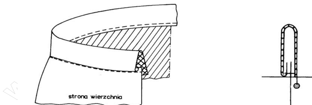
Rysunek 3. Rysunek instruktażowy – wszycie paska do spódnicy
