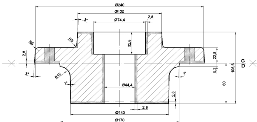
Rysunek surowego odlewu tulei (przykładowe rozwiązanie)
