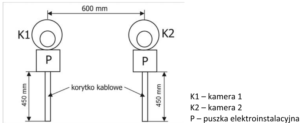
Rysunek 2. Schemat rozmieszczenia kamer, korytek kablowych i puszek elektroinstalacyjnych na płycie montażowej
