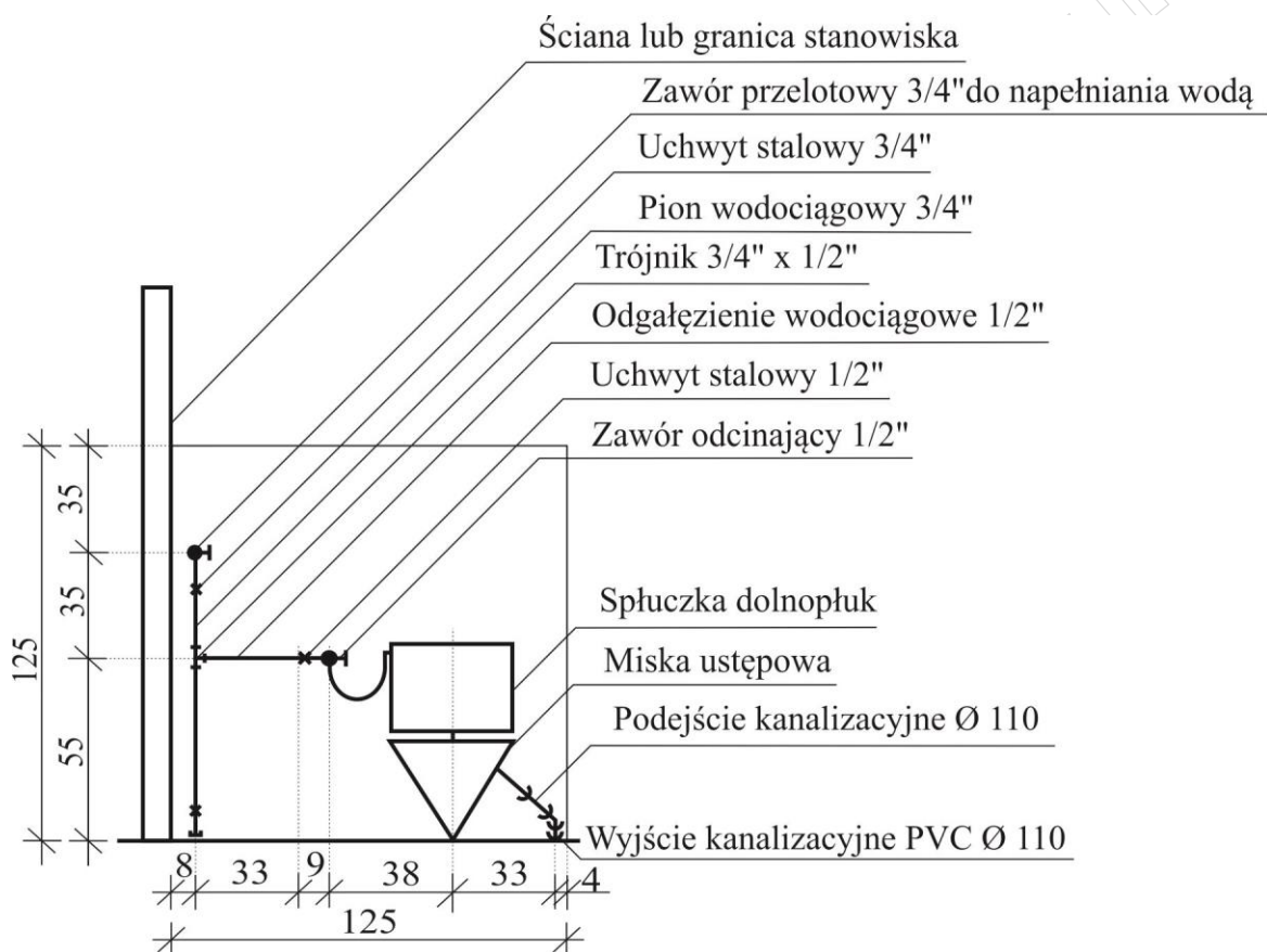
Rysunek 1. Widok instalacji wodociągowej i kanalizacyjnej (wymiary w cm)
