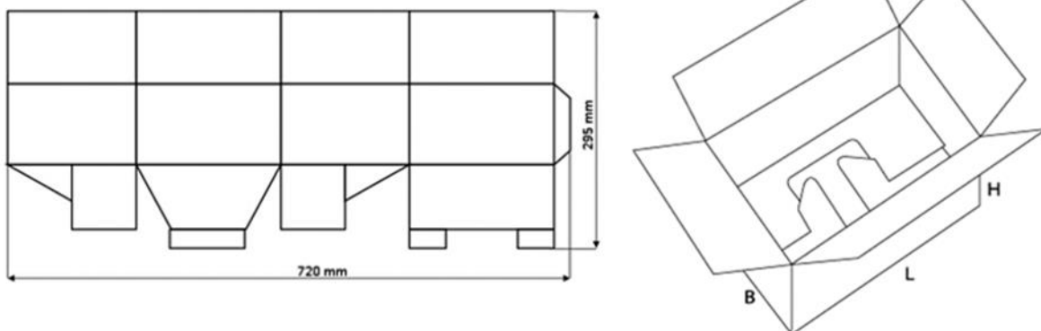
Rysunek 1. Siatka i konstrukcja pudła
